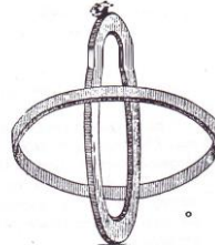
Κρίκος Ισημερινός
