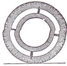
Κρίκος Τροπικός
